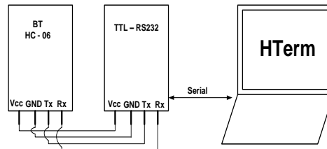
Gambar 4. Konfigurasi Bluetooth HC-06
